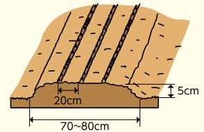
図2 トンネル被覆(穴開きフィルム)
